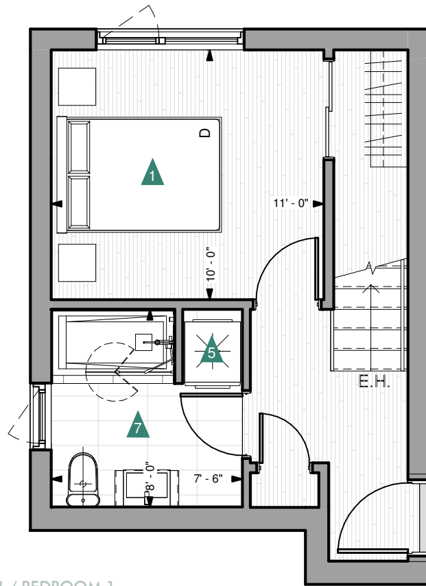
NIV. 2
